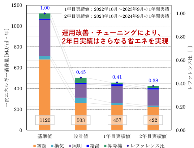
運用段階の ZEB 評価
