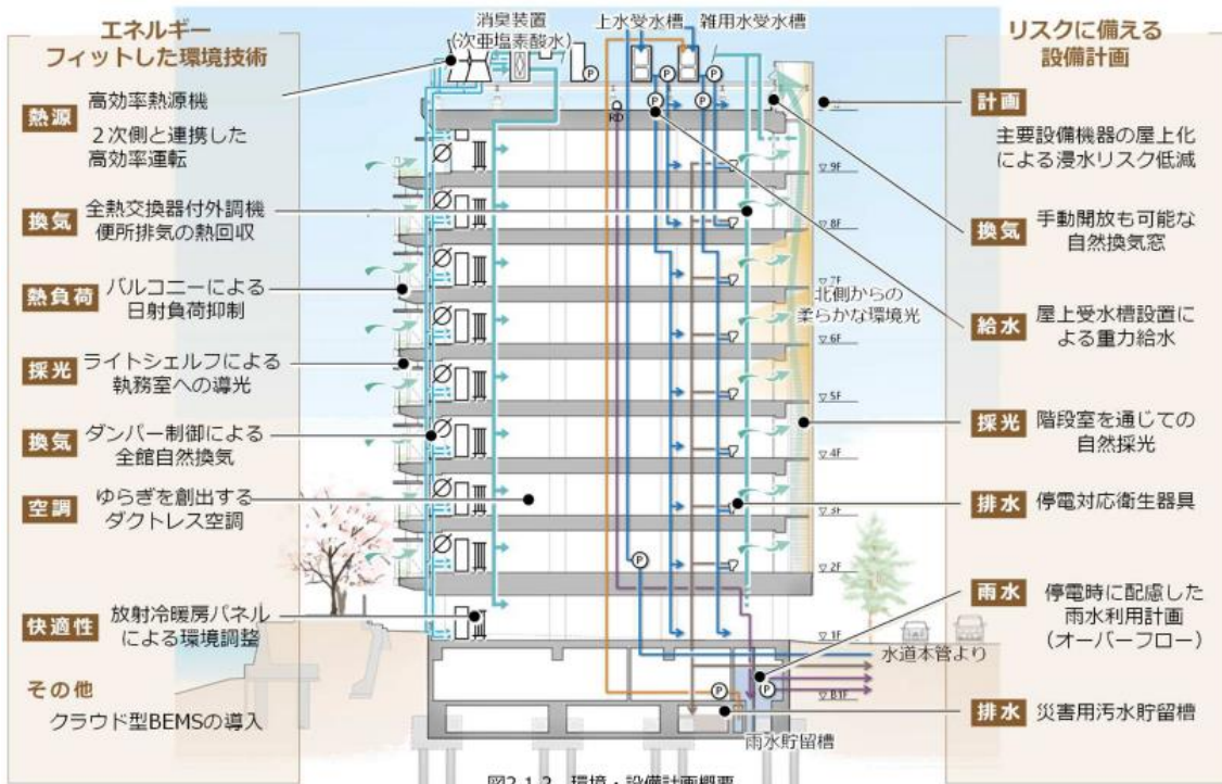
須賀工業本社ビル 環境・設備計画概要
